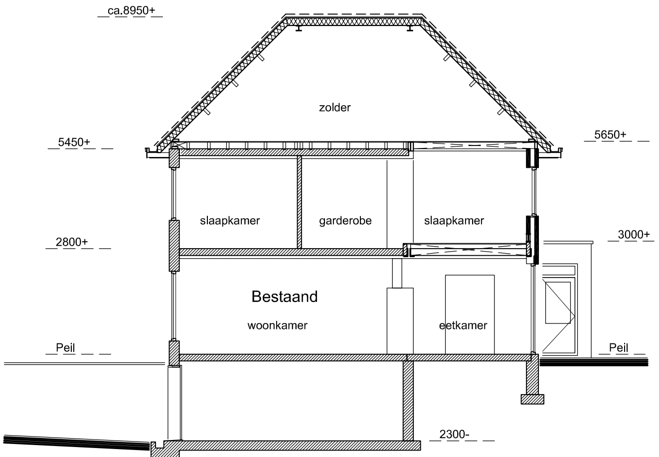
doorsnede nieuw
