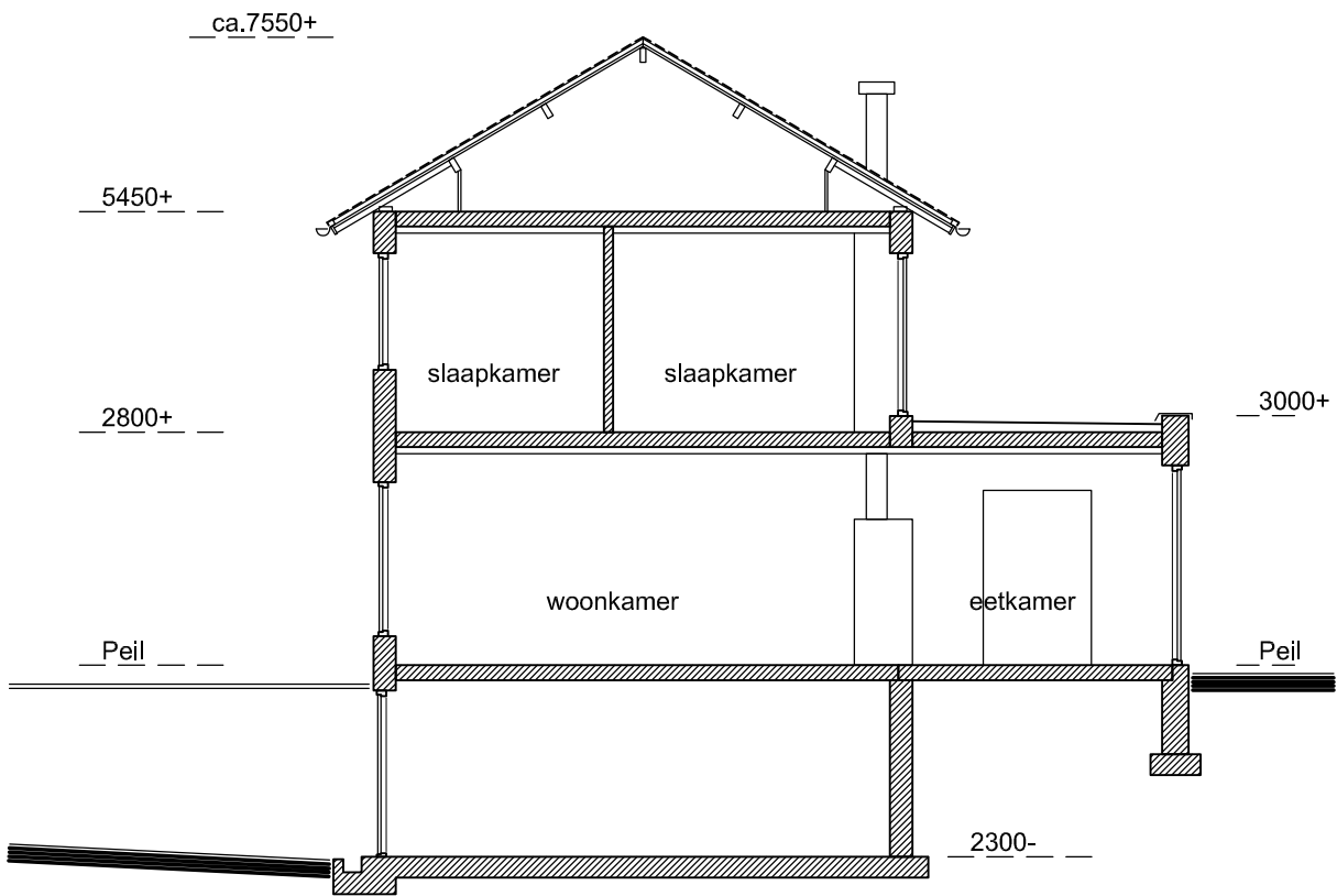
doorsnede bestaand
