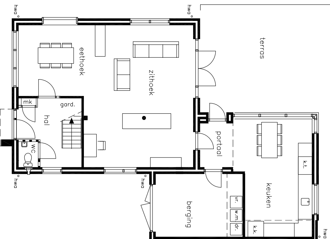
beganegrond Nieuwe toestand
