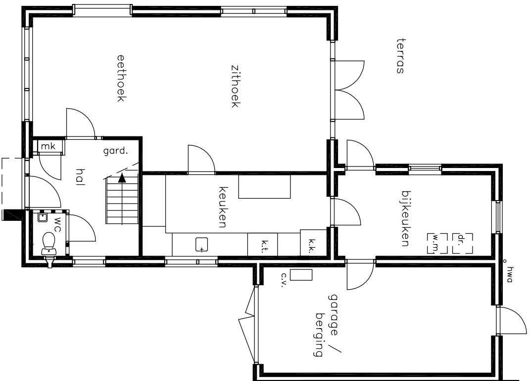
beganegrond Bestaande toestand
